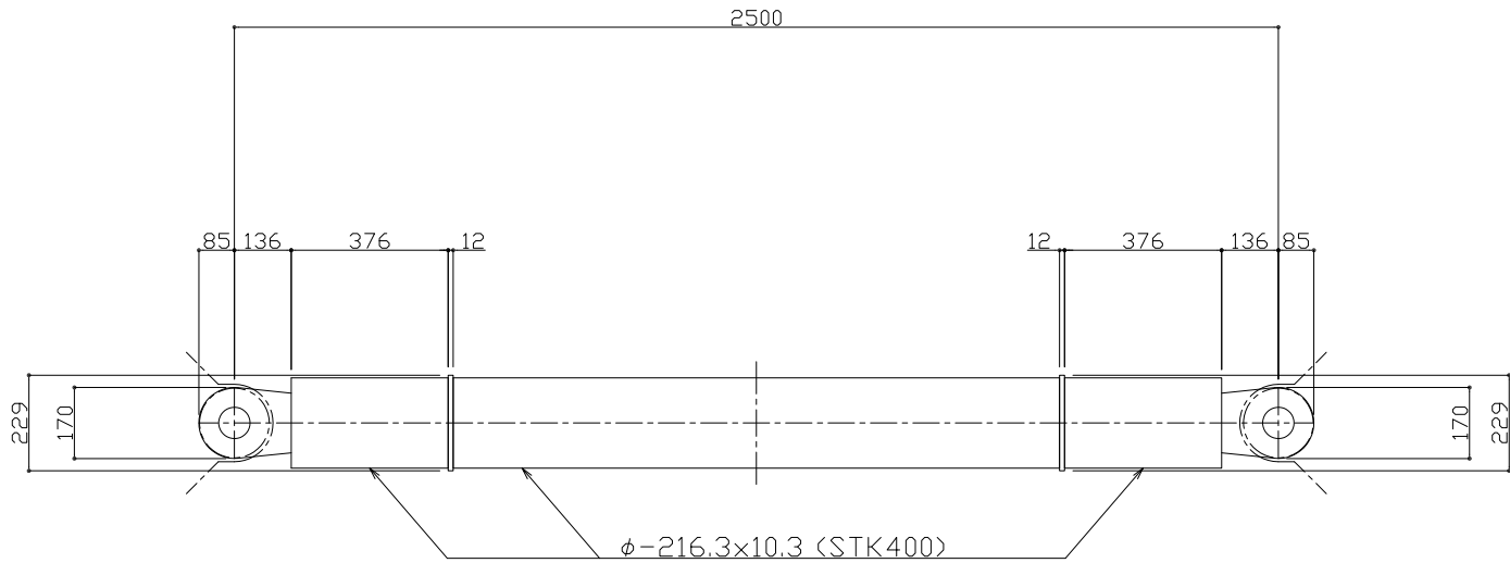
側面図
