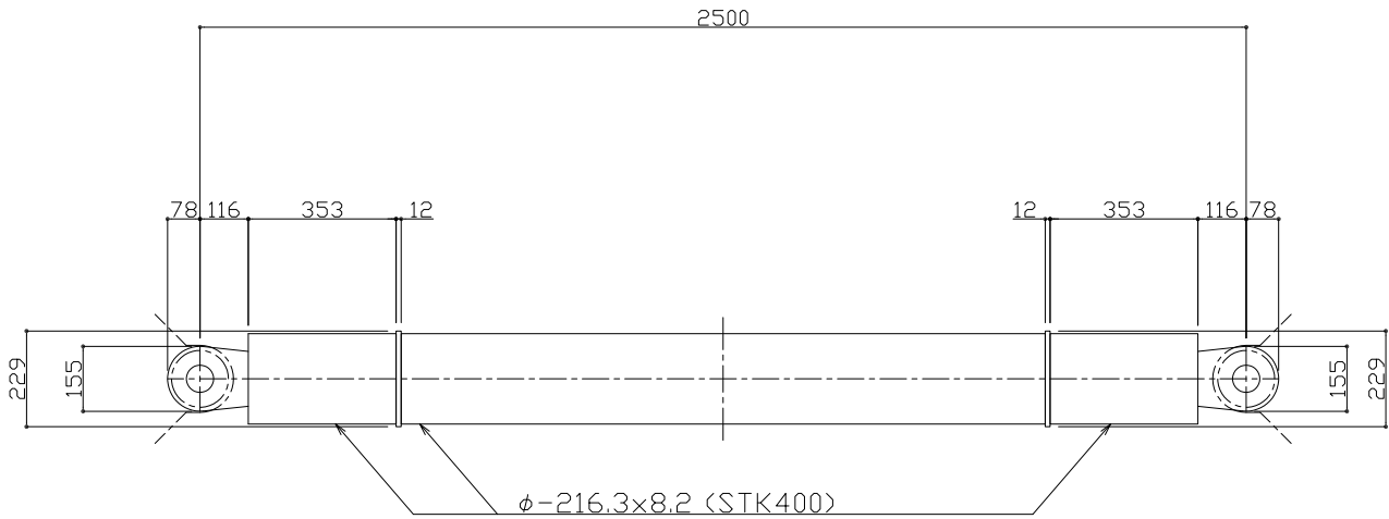
側面図
