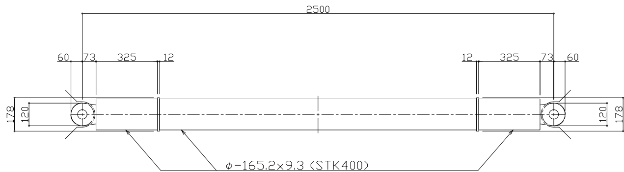
側面図
