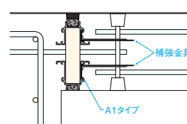
片目地仕様 (A1タイプ)
