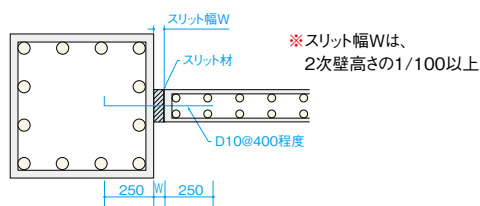
片目地仕様 (A1タイプ)
