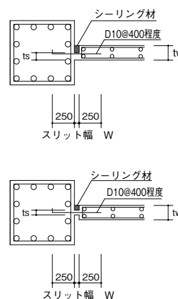
b) 部分スリット型の例
