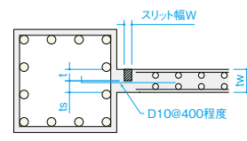
ts= 壁厚 tw の1/2以下、且つ7cm以下。w/ts=0.5~1.0
