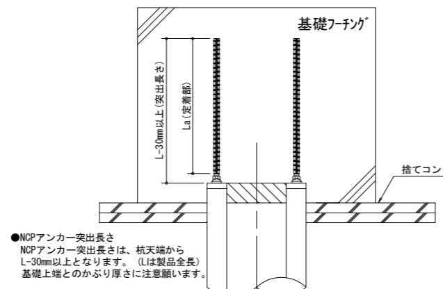
図-6 NCPアンカー工法の一般図
