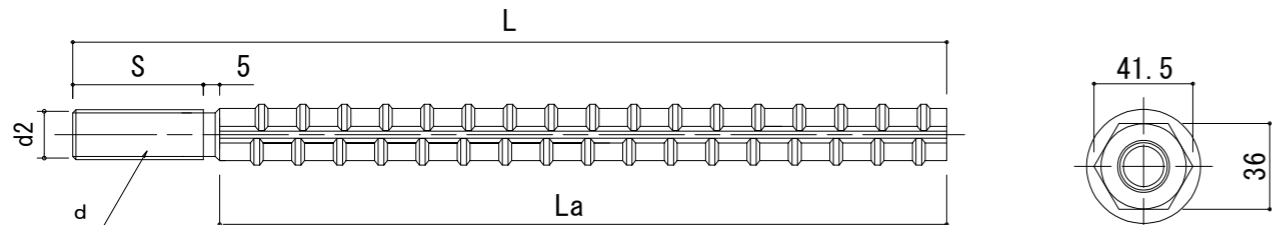
図-1 NCP標準タイプ ボルト形状
