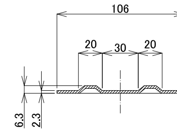
A-A'断面
