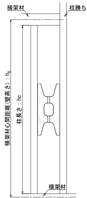
図 3.6 柱勝ちの場合の柱長さ
