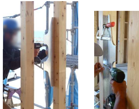
(c) CR2 プレート(OK-65)施工
