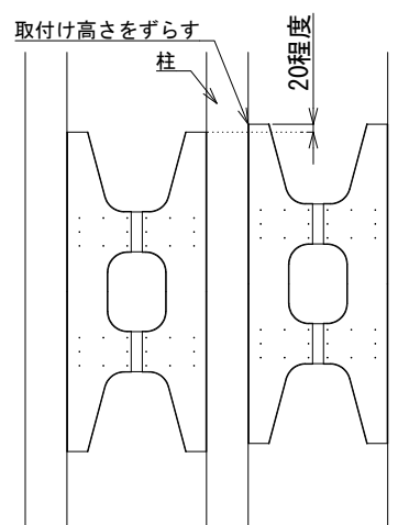
図 3.3 連続した壁に取付ける場合
