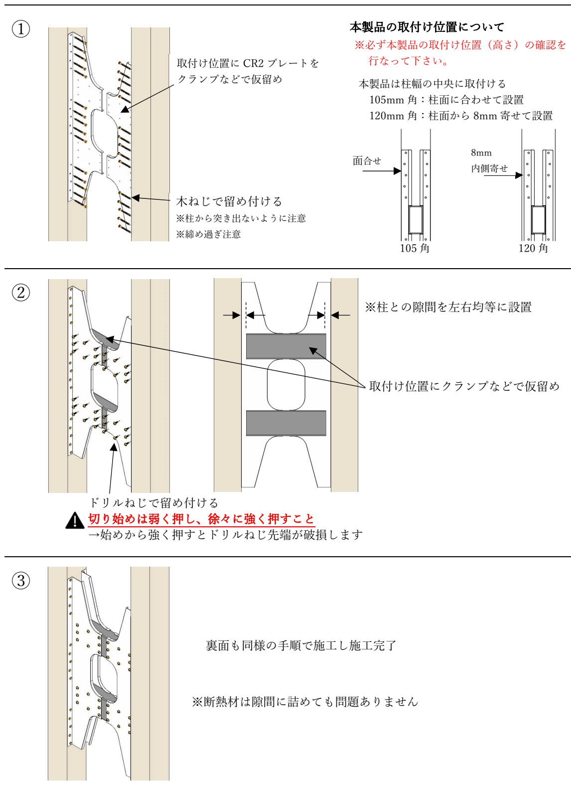
図 4.1 標準的な施工方法
