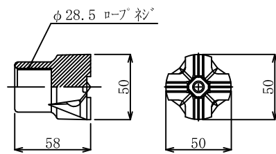
1-a. OSDPチップ付ビット φ50
