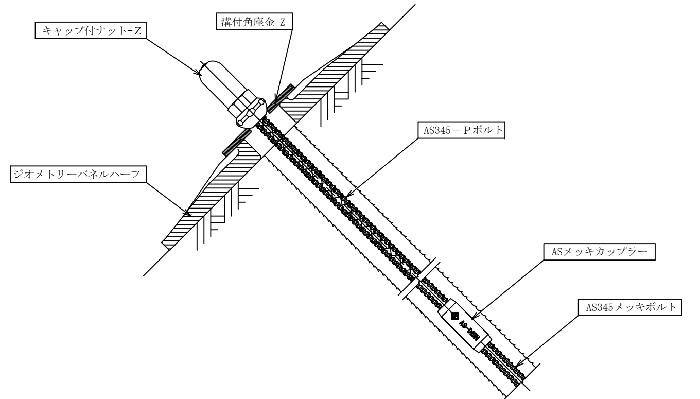
頭部詳細図 1/3
