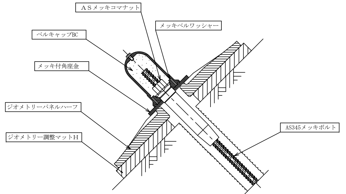
頭部詳細図 1/3
