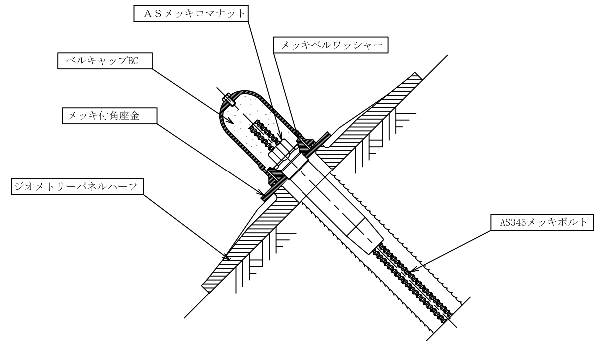
頭部詳細図 1/3
