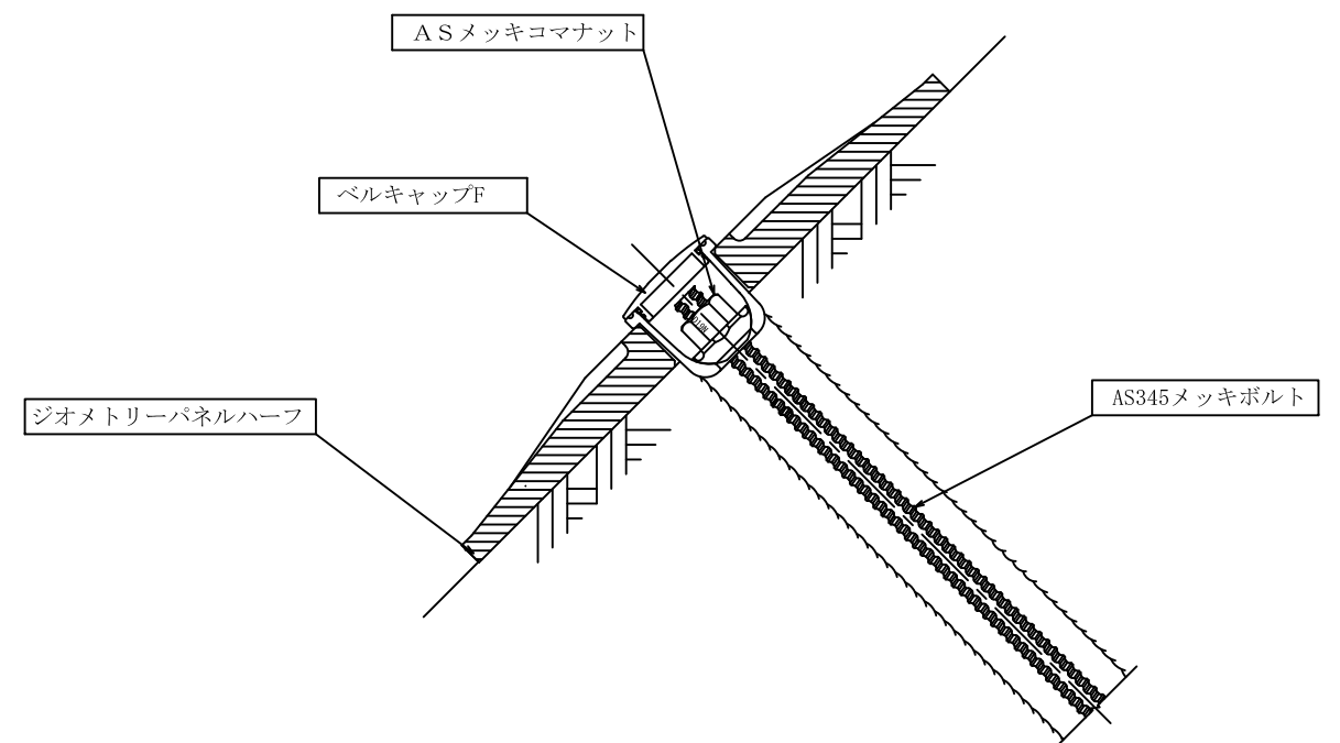
頭部詳細図 1/3
