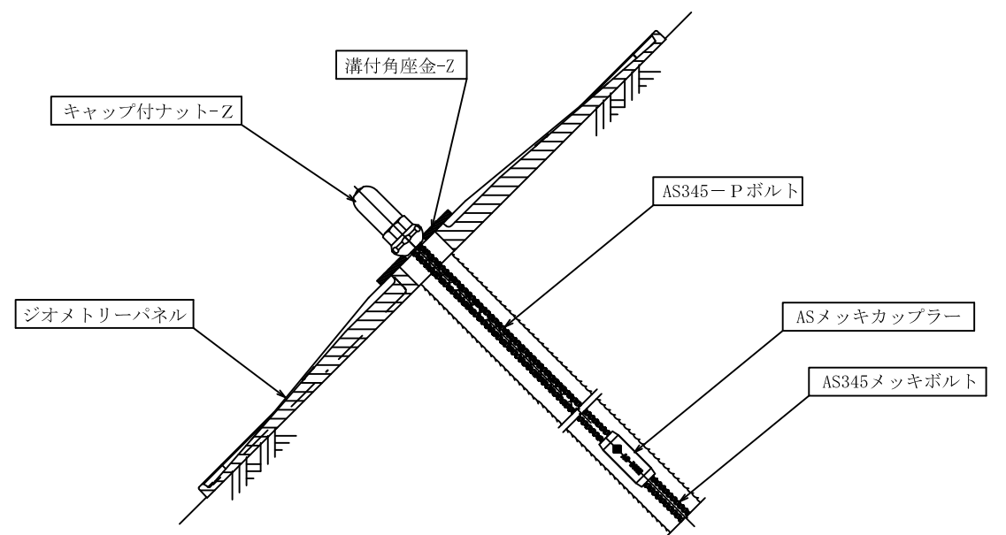
頭部詳細図 1/5
