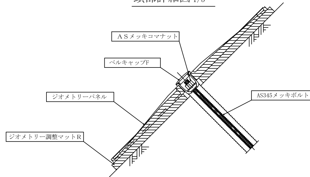
頭部詳細図 1/5
