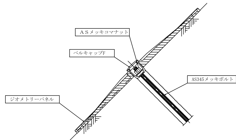
頭部詳細図 1/5
