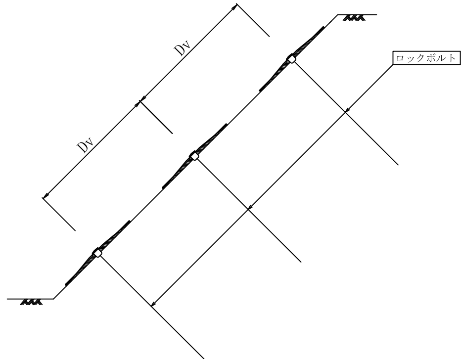
標準断面図 1/20
