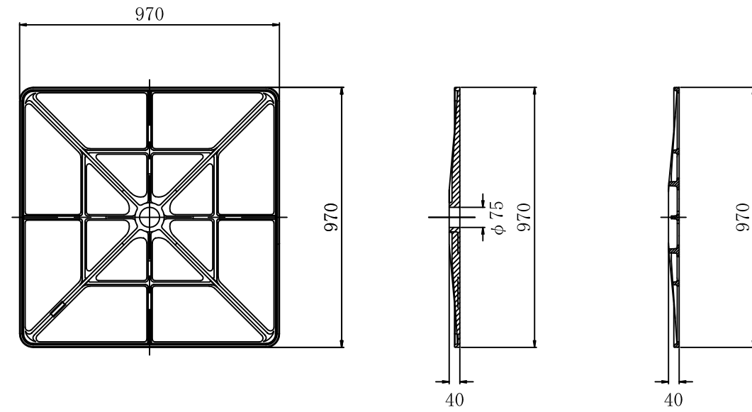
標準構造図 1/10
