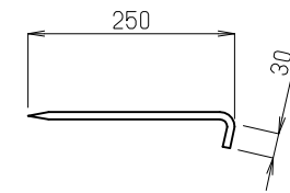
GBピン250 φ9×250×30 詳細図 S=1:10
