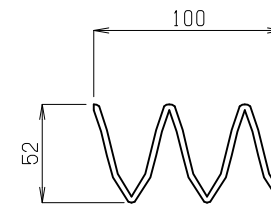
GB連結コイル φ3.2×100×52 詳細図 S=1:4
