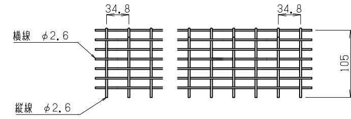
GB枠GB100 正面図 S=1:6
