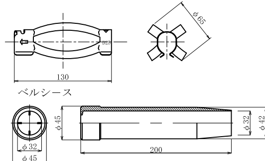
K-1スペーサーD25-65 (電気メッキ)
