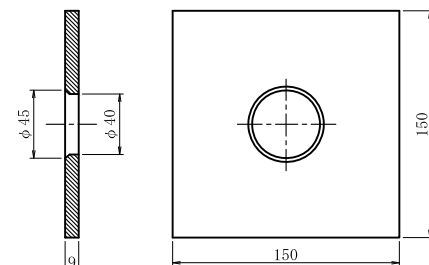
溝付角座金-Z (溶融亜鉛めっき HDZT 77)
