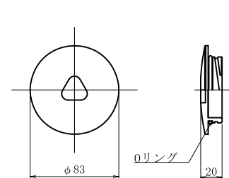
ベルキャップF (蓋部) (溶融亜鉛めっき HDZT 77)
