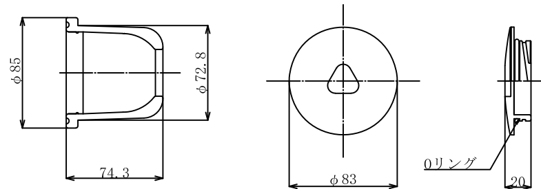
5-1. ベルキャップF (本体) (溶融亜鉛めっき HDZT 77)
