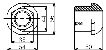
2. ASメッキコマナット D25N (溶融亜鉛めっき HDZT 49)
