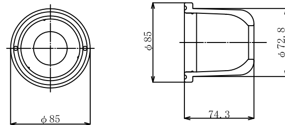
6-1. ベルキャップF (本体) (溶融亜鉛めっき HDZT 77)
