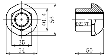
2. ASメッキコマナット D22NT (溶融亜鉛めっき HDZT 49)
