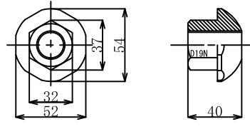
2. ASメッキコマナット D19N (溶融亜鉛めっき HDZT 49)
