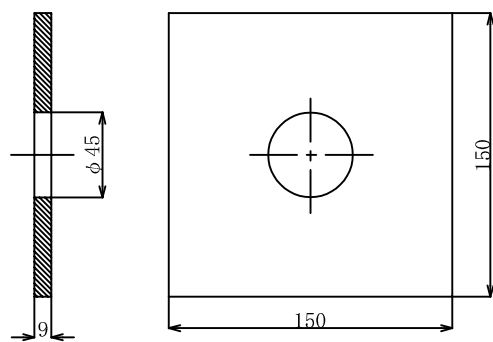
4. 角座金
