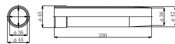
4. ベルシース (D29・32用)
