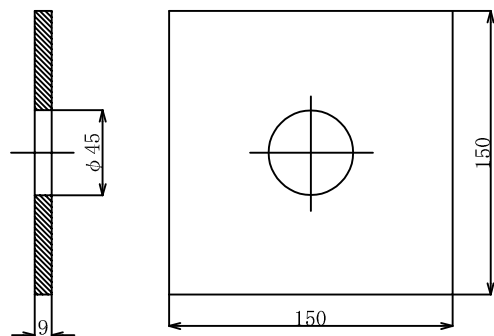
5. 角座金
