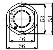
2. ASコマナット (D29N用)
