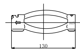
4. K-1スペーサーD25-65 (電気メッキ)
