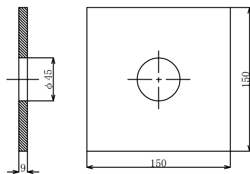
5. 角座金
