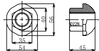
2. ASコマナット D22N
