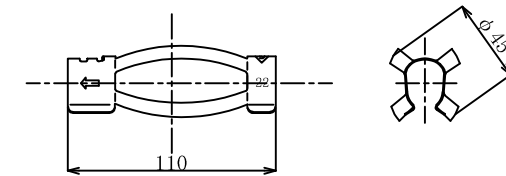
4. K-1スペーサーD22-45 (電気メッキ)
