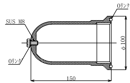
7. ボルトキャップBC
