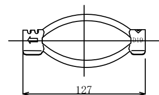
4. K-1スペーサーD19-65 (電気メッキ)
