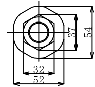
2. ASメッキコマナット D19N (溶融亜鉛めっき HDZT 49)
