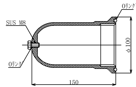
8. ベルキャップBC
