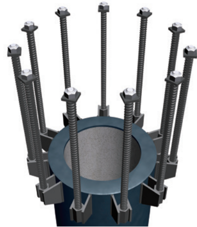
設置本数上限の例 (φ700 D38-M 11本)
