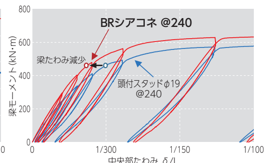
梁中央部曲げモーメント-たわみ関係 (実大梁曲げ実験)
