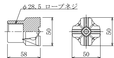
1-a. OSDPチップ付ビット φ50
