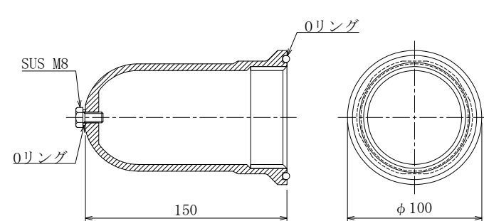
7. ベルキャップBC
