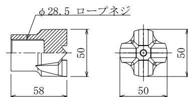
1-b. OSDP鉄ビット φ50
