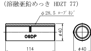
OSDPメッキカップラーR (溶融亜鉛めっき HDZT 77)
