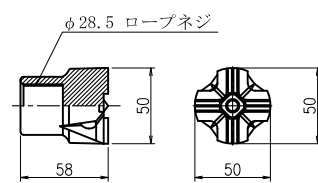
溝付角座金-Z (溶融亜鉛めっき HDZT 77)
