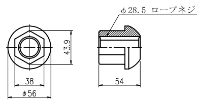
OSDPメッキナット (溶融亜鉛めっき HDZT 49)
