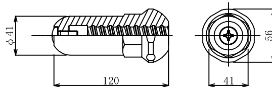
2. キャップ付ナット D22NT-Z (溶融亜鉛めっき HDZT 49)
