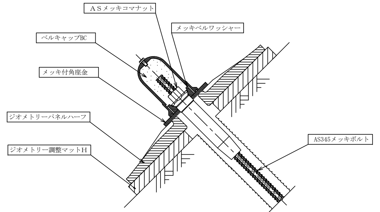
頭部詳細図 1/3
