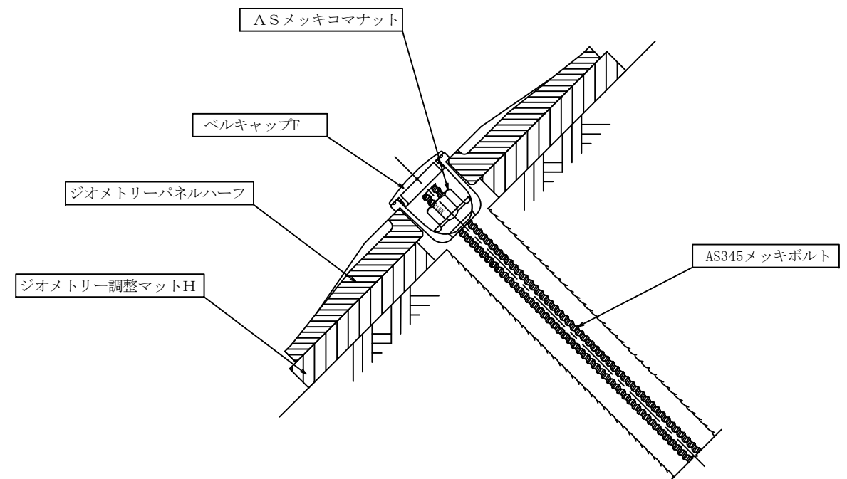
頭部詳細図 1/3
