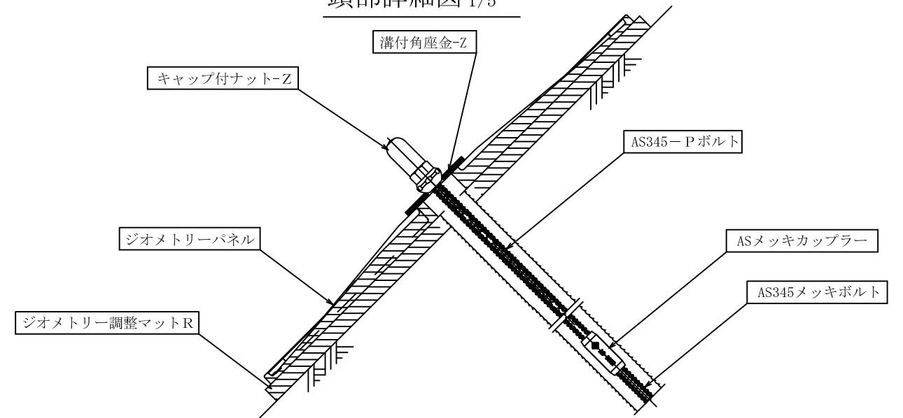
頭部詳細図 1/5
