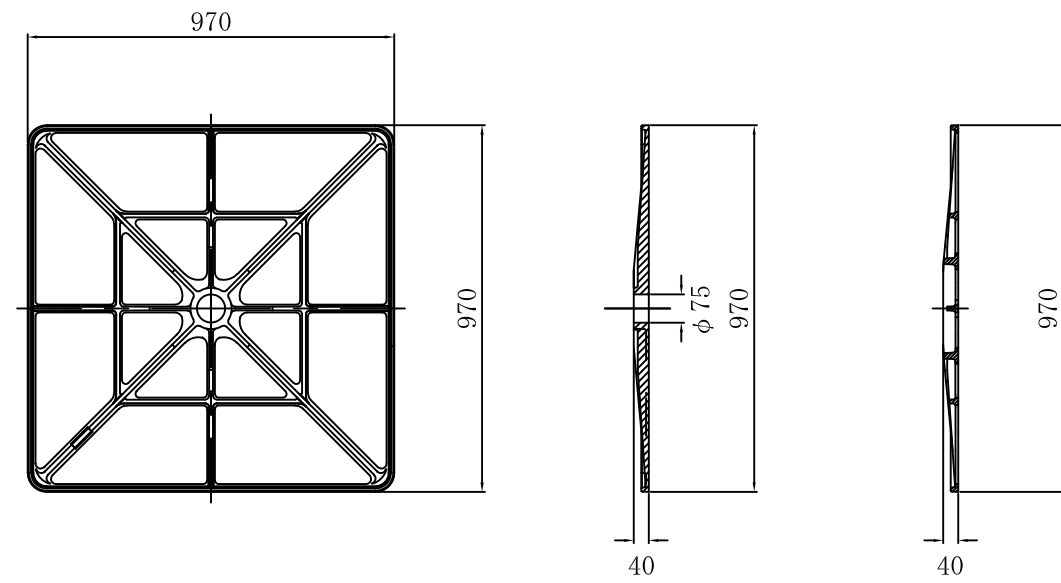
標準構造図 1/10
