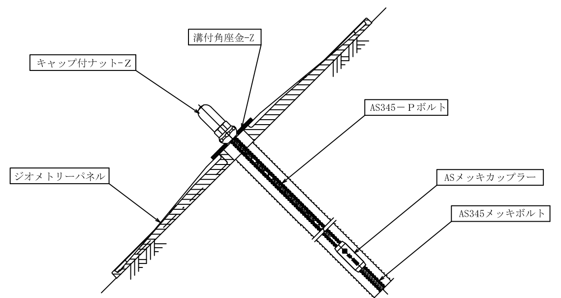
頭部詳細図 1/5
