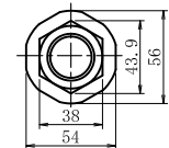
ASメッキコマナット D25N (溶融亜鉛めっき HDZT 49)
