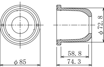
ベルキャップF (本体) (溶融亜鉛めっき HDZT 77)
