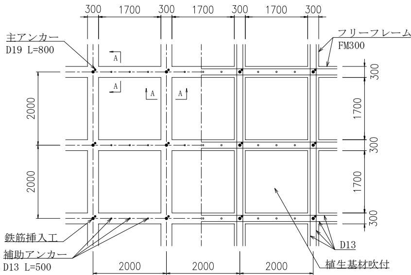
展開図 S=1/100
