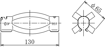
K-1スペーサー D25-65 (電気めっき)
