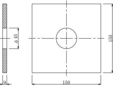
メッキ付角座金 (溶融亜鉛めっき HDZT 77)
