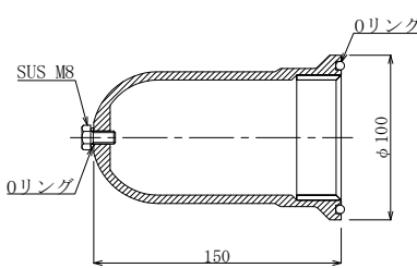
ベルキャップBC
