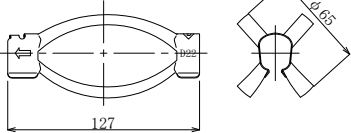
K-1スペーサー D22-65 (電気めっき)
