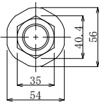
ASメッキコマナット D22NT (溶融亜鉛めっき HDZT 49)
