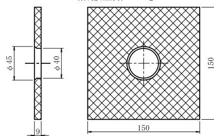
角座金-P (溶融亜鉛めっき HDZT 77+PVB樹脂)
