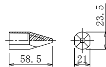
メッキ付角座金 (溶融亜鉛めっき HDZT 77)
