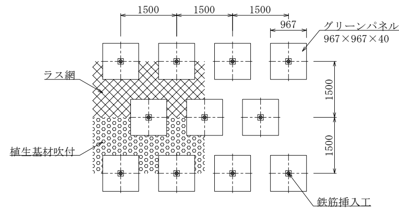
展開図 S=1/100
