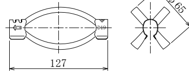
ベルキャップF (本体) (溶融亜鉛めっき HDZT 77)
