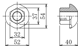
ASメッキコマナット D19N (溶融亜鉛めっき HDZT 49)
