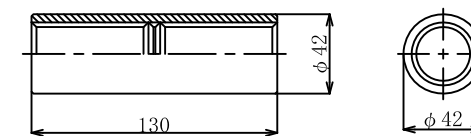
4. AS29NメッキカップラーZ (溶融亜鉛めっき HDZT 77)
