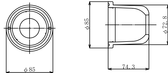
6-1. ベルキャップF (本体) (溶融亜鉛めっき HDZT 77)
