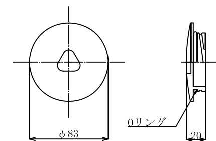
5-2. ベルキャップF (蓋部) (溶融亜鉛めっき HDZT 77)
