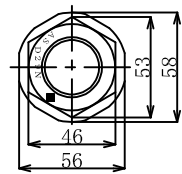
2. ASメッキコマナット D29N (溶融亜鉛めっき HDZT 49)
