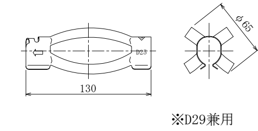
3. K-1スパーサー D25-65 (電気めっき)
