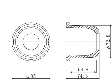
5-1. ベルキャップF (本体) (溶融亜鉛めっき HDZT 77)
