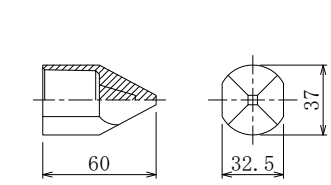
1. 先端キャップ D29
