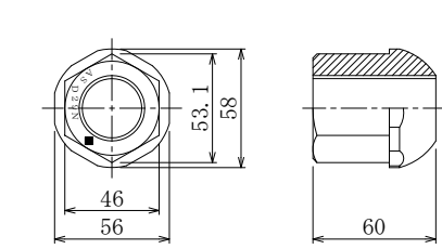
2. ASメッキコマナット D29N (溶融亜鉛めっき HDZT 49)
