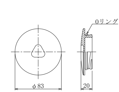
5-2. ベルキャップF (蓋部) (溶融亜鉛めっき HDZT 77)
